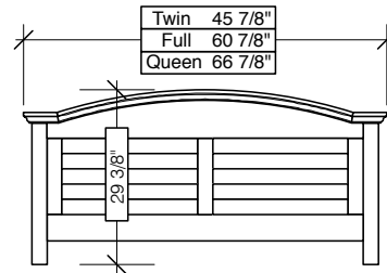
SANDPIPER FOOTBOARD
